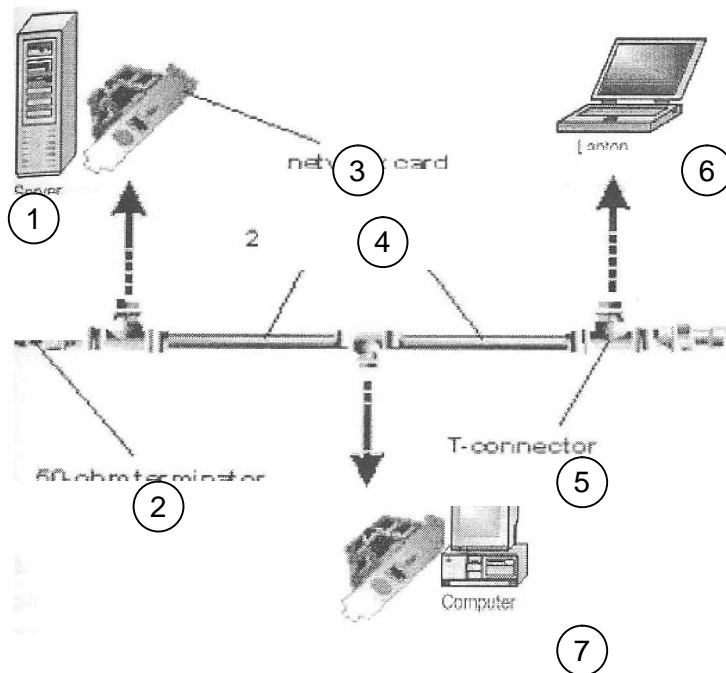
Gambar 17. Gambaran Pemasangan Kabel Coaxial dengan Konektor BNC pada Jaringan dengan Topologi Bus
