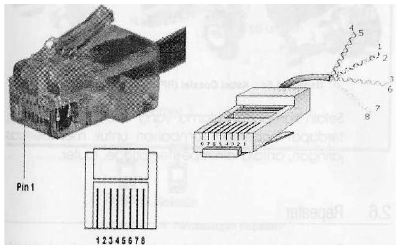
Gambar 9. Susunan Konektor dan Pengkabelannya
