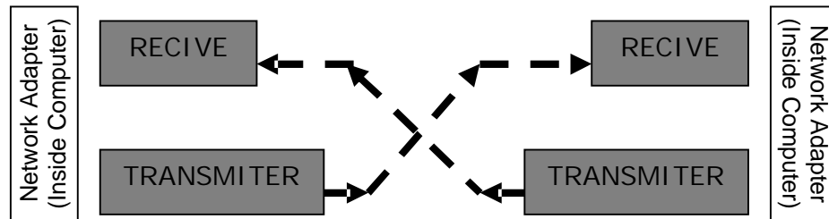
Gambar 16. Pengiriman dan Penerimaan Data pada Kabel Silang (Crossover Cable)
