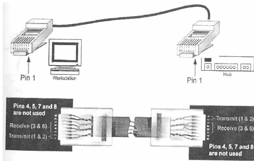
Gambar 27. Pengiriman Data dengan Model Kabel Lurus
