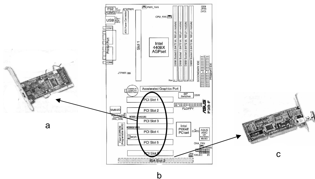
Gambar 10. Pemasangan Kartu Jaringan pada Motherboard
