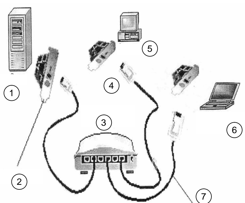
Gambar 18. Gambaran Pemasangan Kabel UTP dengan Konektor RJ 45 pada Jaringan dengan Topologi Star
